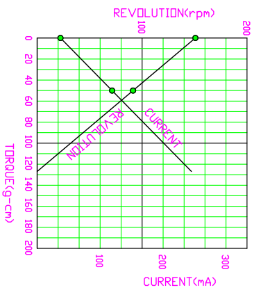
8GL-3S T-N特性
